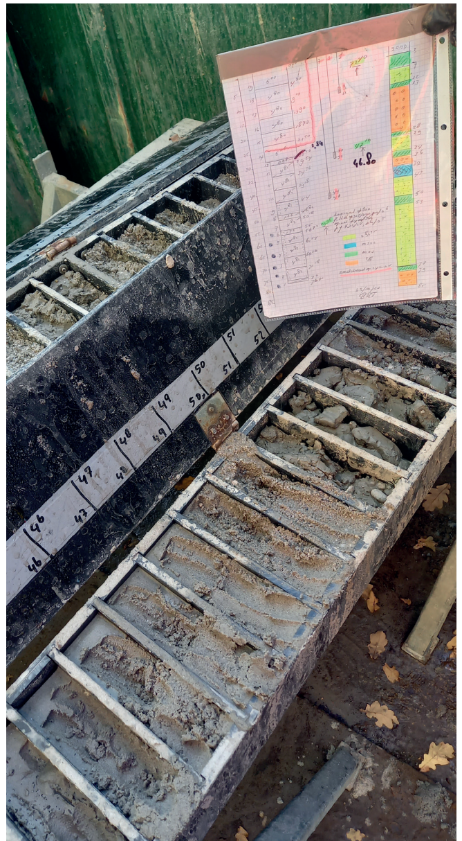
Afb. 4: Elke meter wordt er een grondmonster genomen, op basis hiervan weet Jan hoe de grond is opgebouwd en hoe hij later de boorgang weer aan moet vullen.
